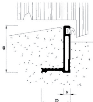
Coupe verticale sur Ouvrant
